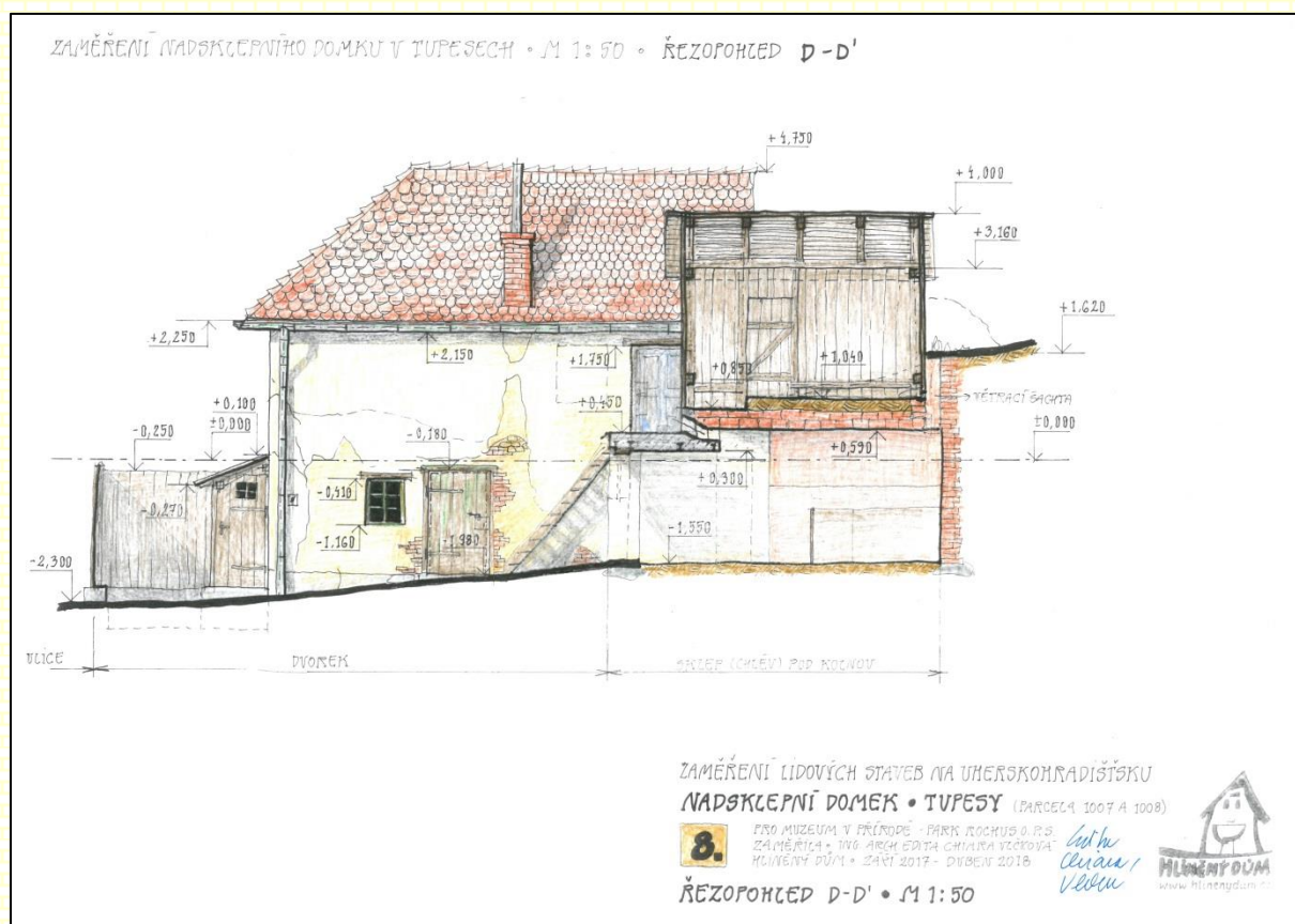
Jeden z výkresů architektonicko-stavební dokumentace nadsklepního domku z Tupes
