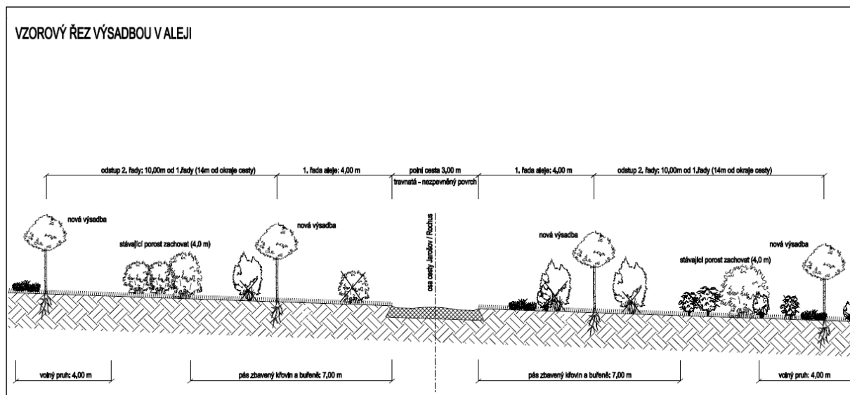
Obr. č. 9: Návrh řešení alejí
