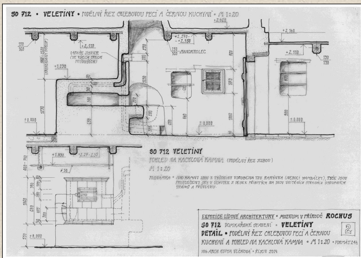
Obr. č. 5: Podélný řez chlebovou pecí a černou kuchyní v expozičním objektu Veletiny č. p. 25
